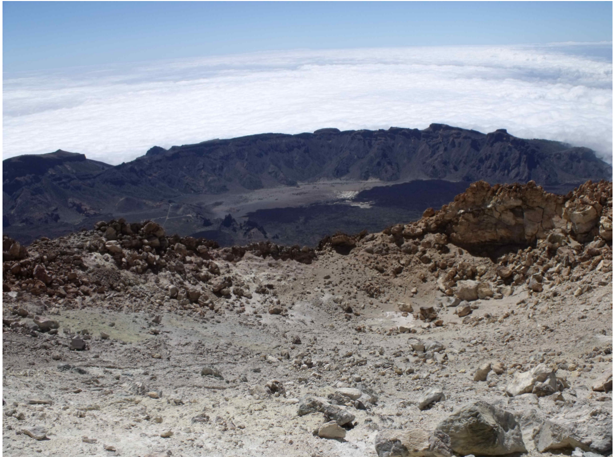
Teidekrater, tief unten der Llano de Ucanca und der Kraterrand der Canadas
